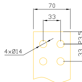
DETAIL VÝVODŮ NN DETAIL VÝVODŮ VN
