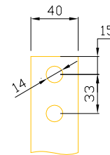
DETAIL VÝVODŮ NN
