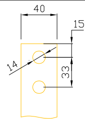
DETAIL VÝVODŮ NN
