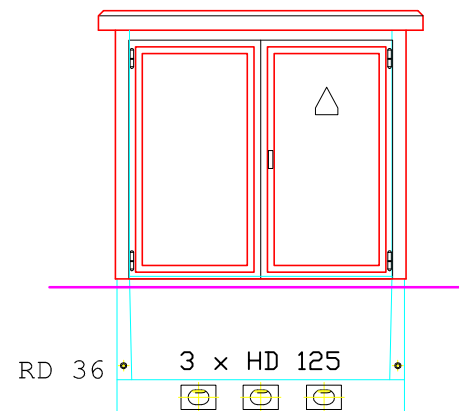
Pohled D
