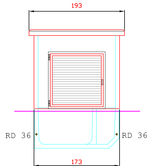
Pohled B
