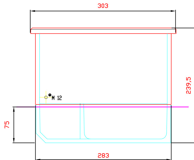
Pohled A
