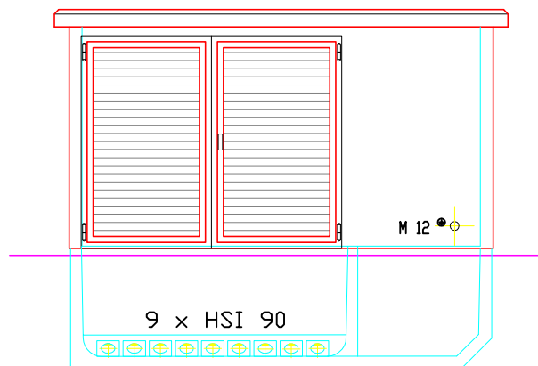
Pohled C
