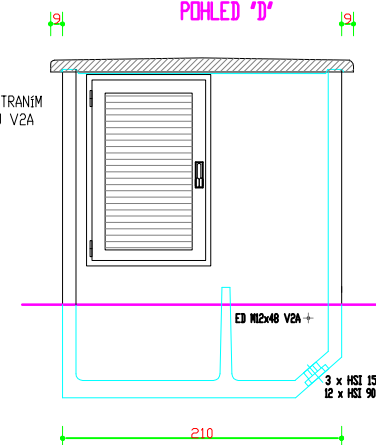
POHLED 'D'
