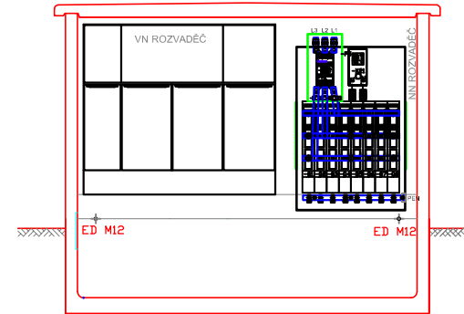
REZ 'B - B'
