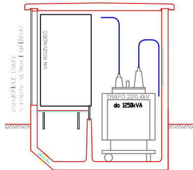
REZ 'C - C'
