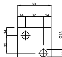
NN Praporec Materiál: Hliník (60x5)
